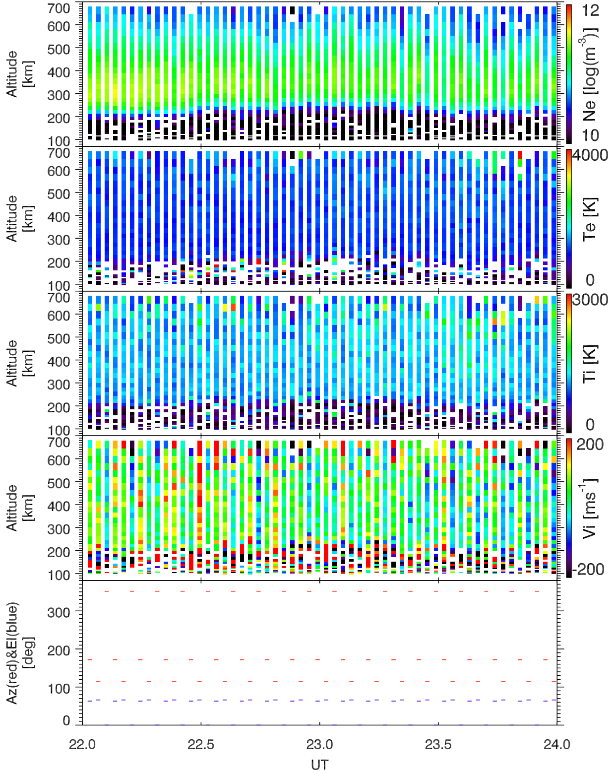
EISCAT 2002-11-14_22_24UT_tau0_ant@32m.
