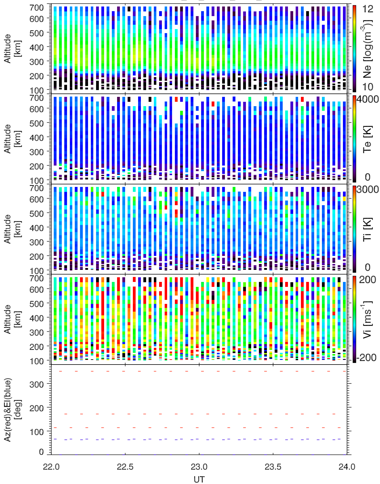
EISCAT 2003-01-07_22_24UT_tau0_ant@32m.
