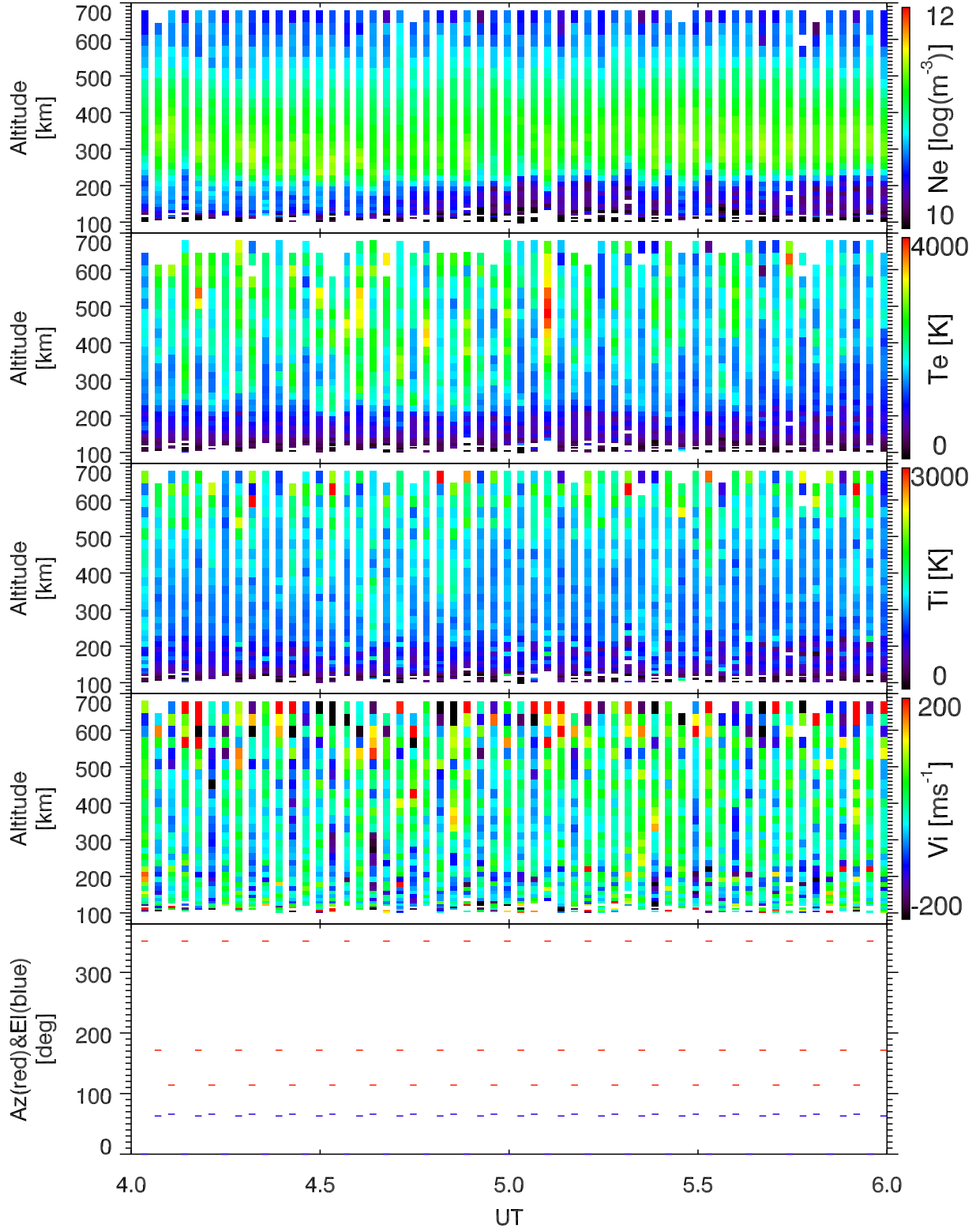
EISCAT 2003-01-08_04_06UT_tau0_ant@32m.
