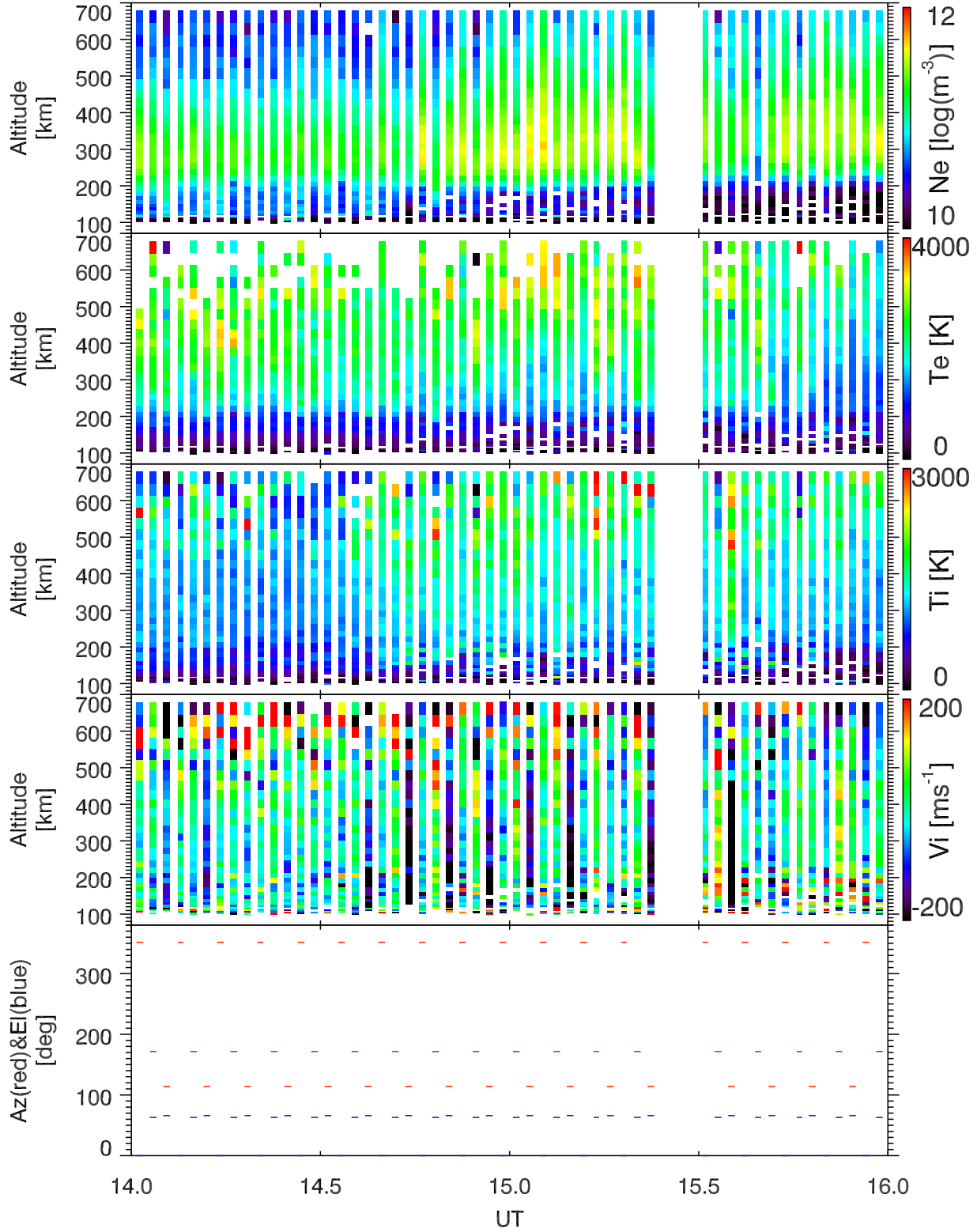
EISCAT 2003-02-12_14_16UT_tau0_all@32m.
