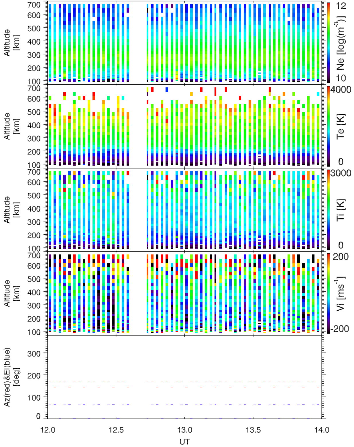
EISCAT 2003-03-19_12_14UT_tau0_ant@32m.
