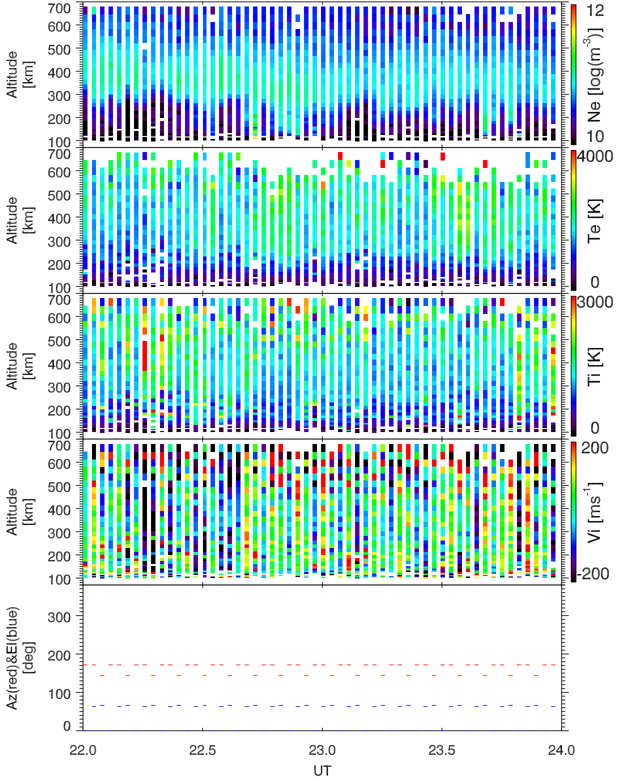
EISCAT 2003-03-19_22_24UT_tau0_ant@32m.
