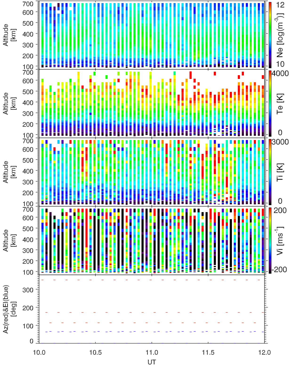
EISCAT 2003-03-21_10_12UT_tau0_ant@32m.
