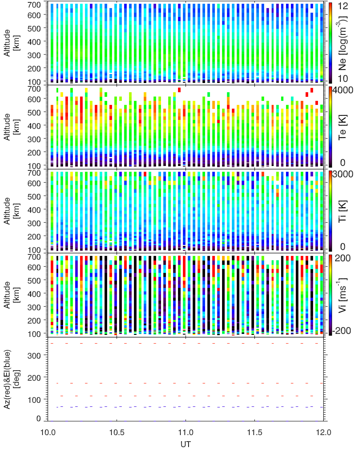
EISCAT 2003-03-22_10_12UT_tau0_ant@32m.
