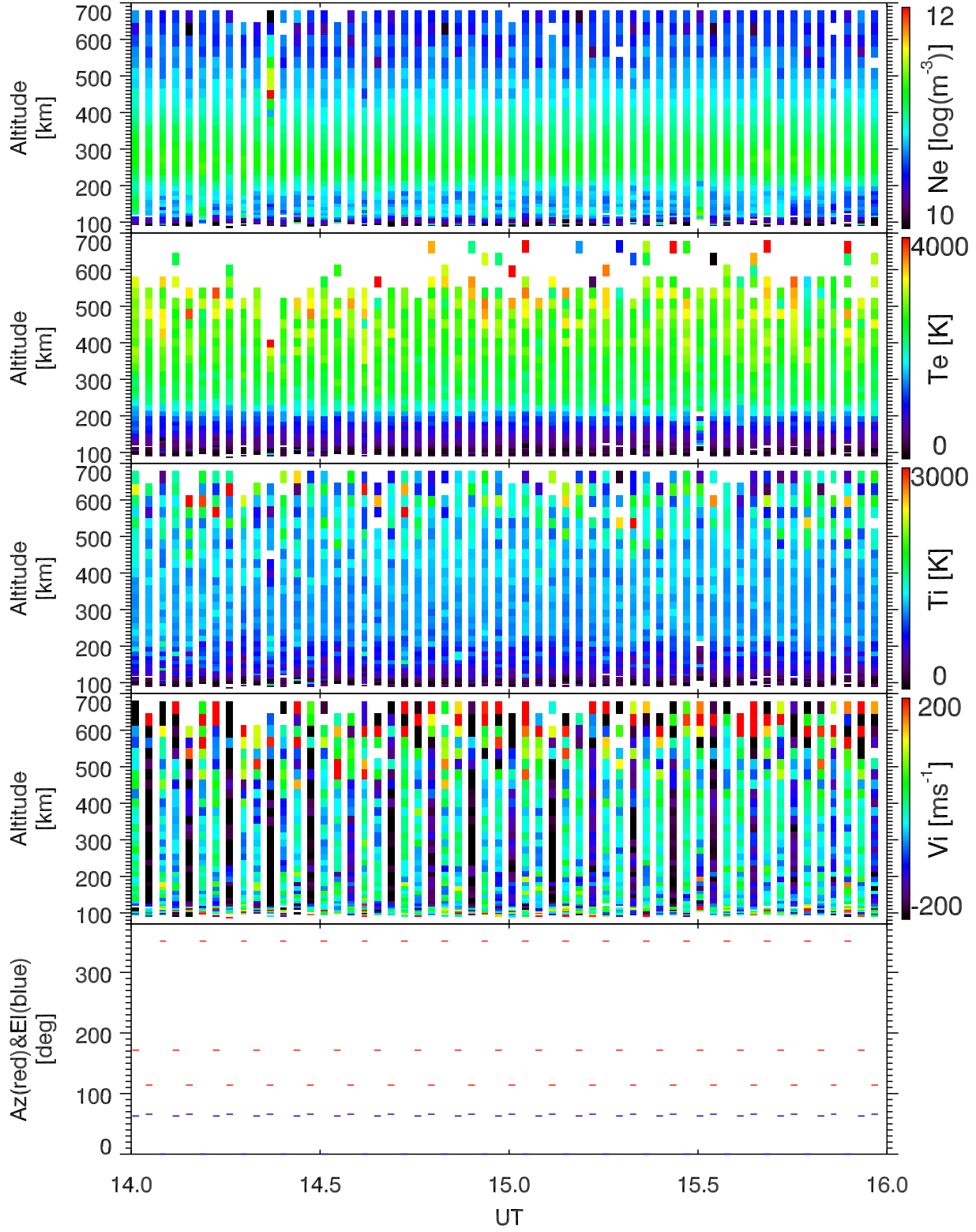
EISCAT 2003-03-22_14_16UT_tau0_ant@32m.
