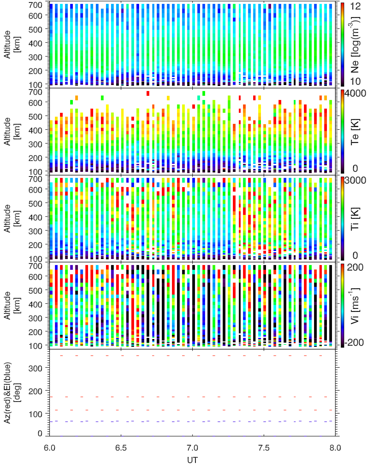
EISCAT 2003-03-23_06_08UT_tau0_ant@32m.
