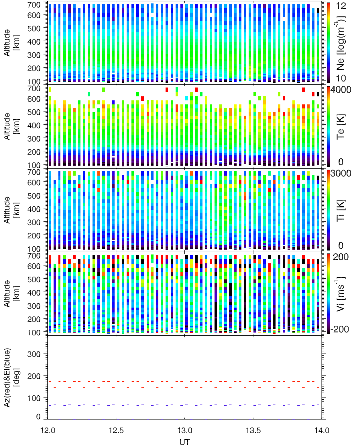
EISCAT 2003-03-23_12_14UT_tau0_ant@32m.
