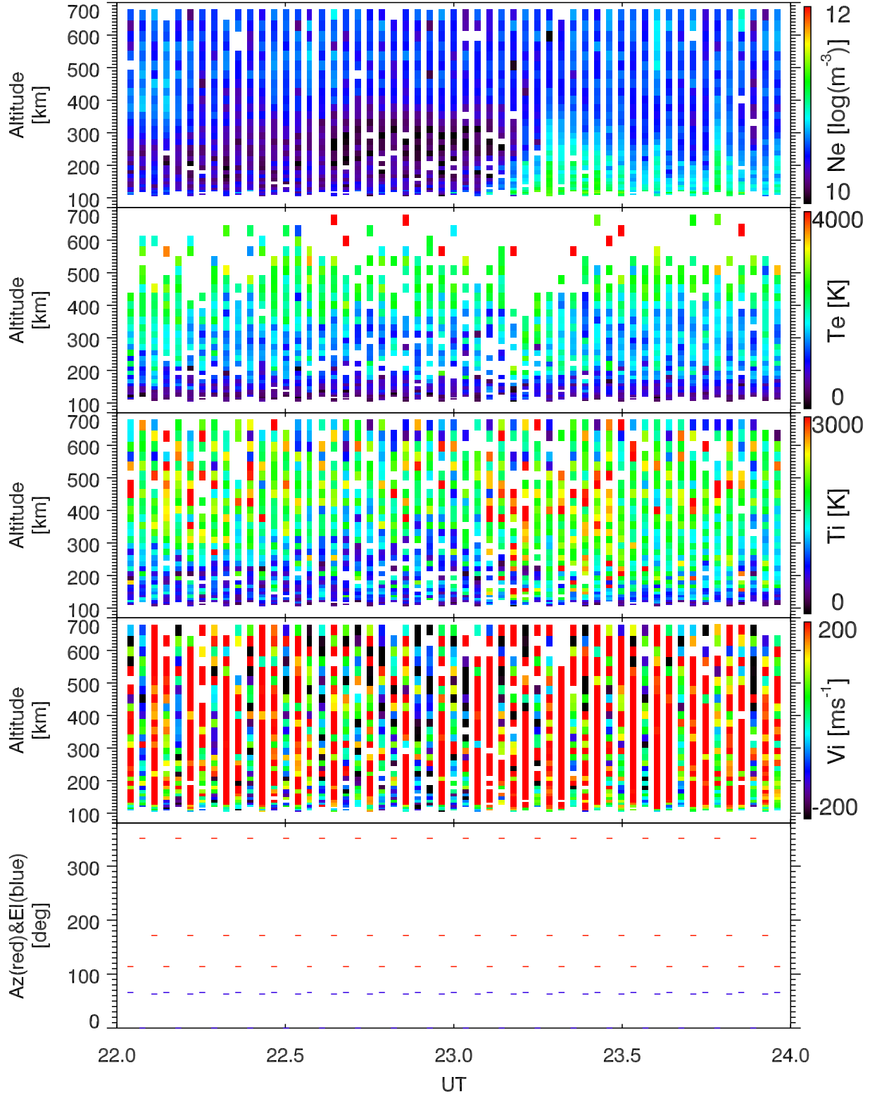
EISCAT 2003-10-29_22_24UT_tau0_ant@32m.
