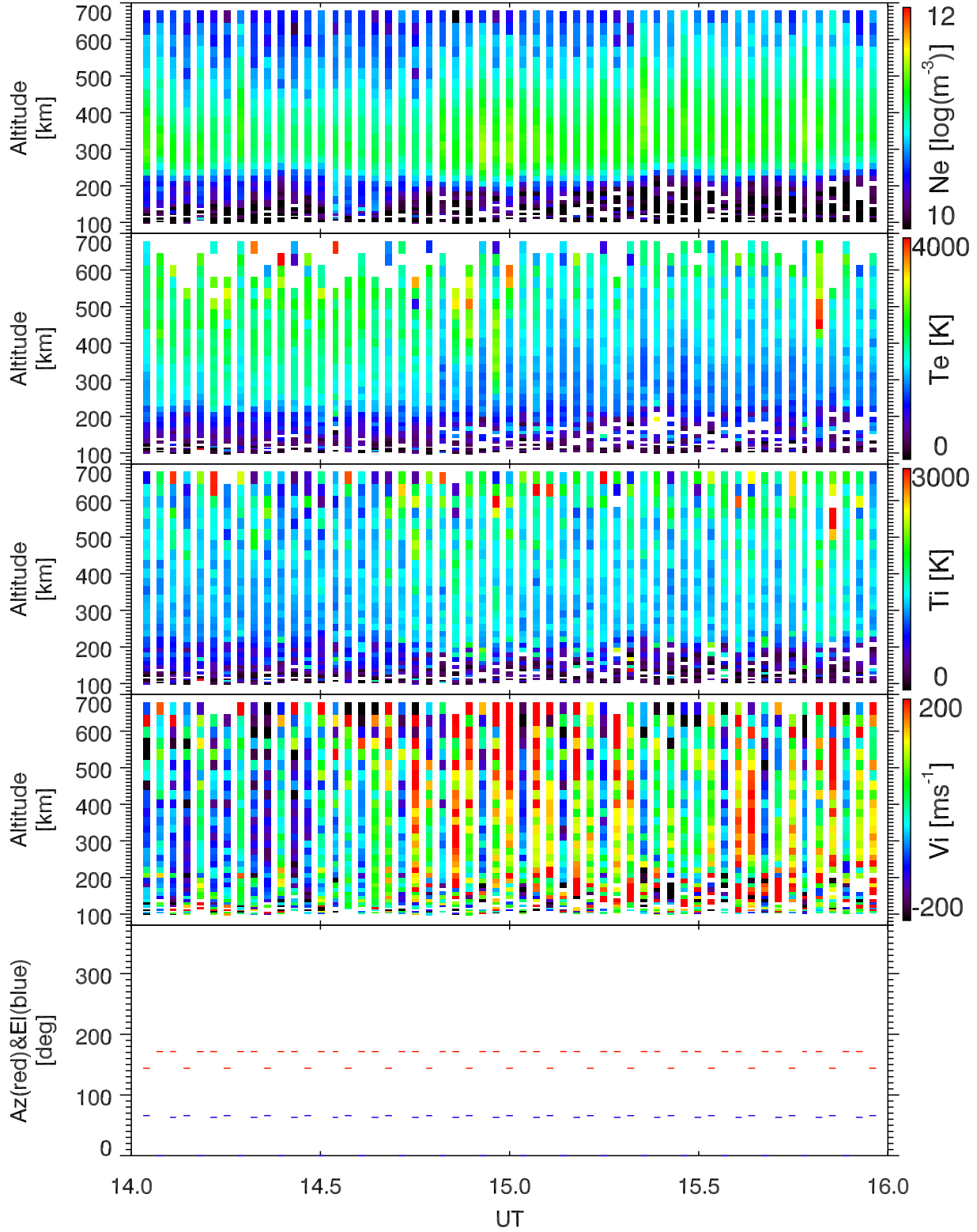
EISCAT 2003-11-01_14_16UT_tau0_ant@32m.
