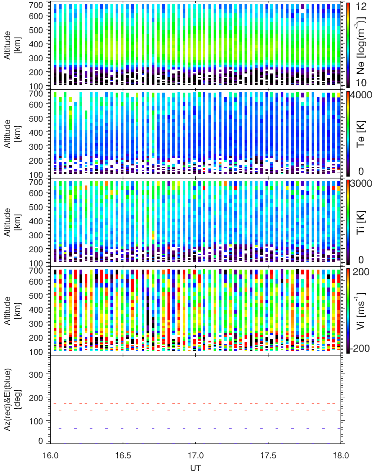
EISCAT 2003-11-01_16_18UT_tau0_ant@32m.
