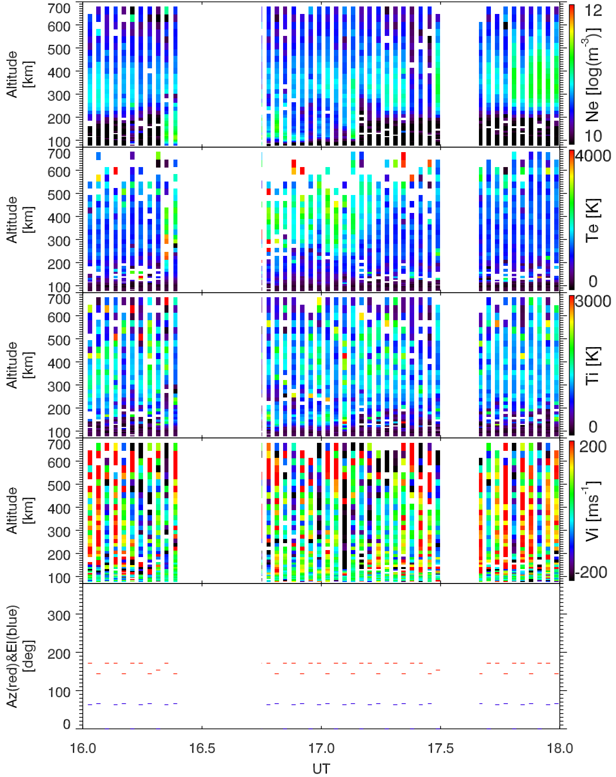
EISCAT 2003-11-12_16_18UT_steffe_ant@32m.
