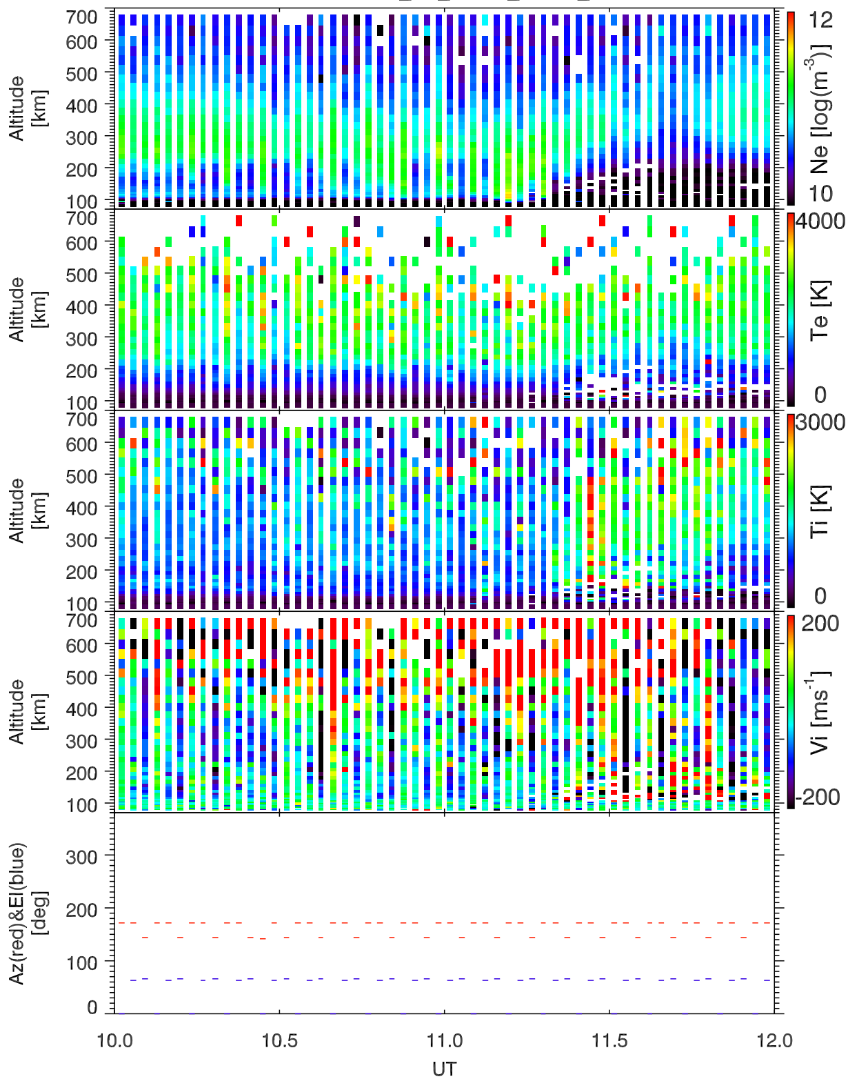
EISCAT 2003-11-13_10_12UT_steffe_ant@32m.
