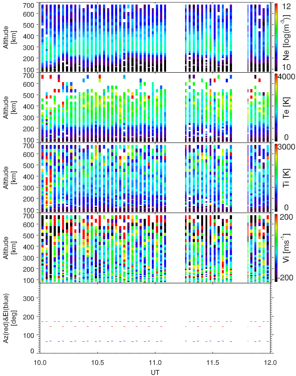
EISCAT 2003-11-14_10_12UT_steffe_ant@32m.
