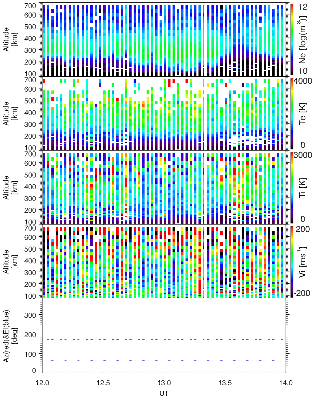
EISCAT 2003-11-16_12_14UT_steffe_ant@32m.
