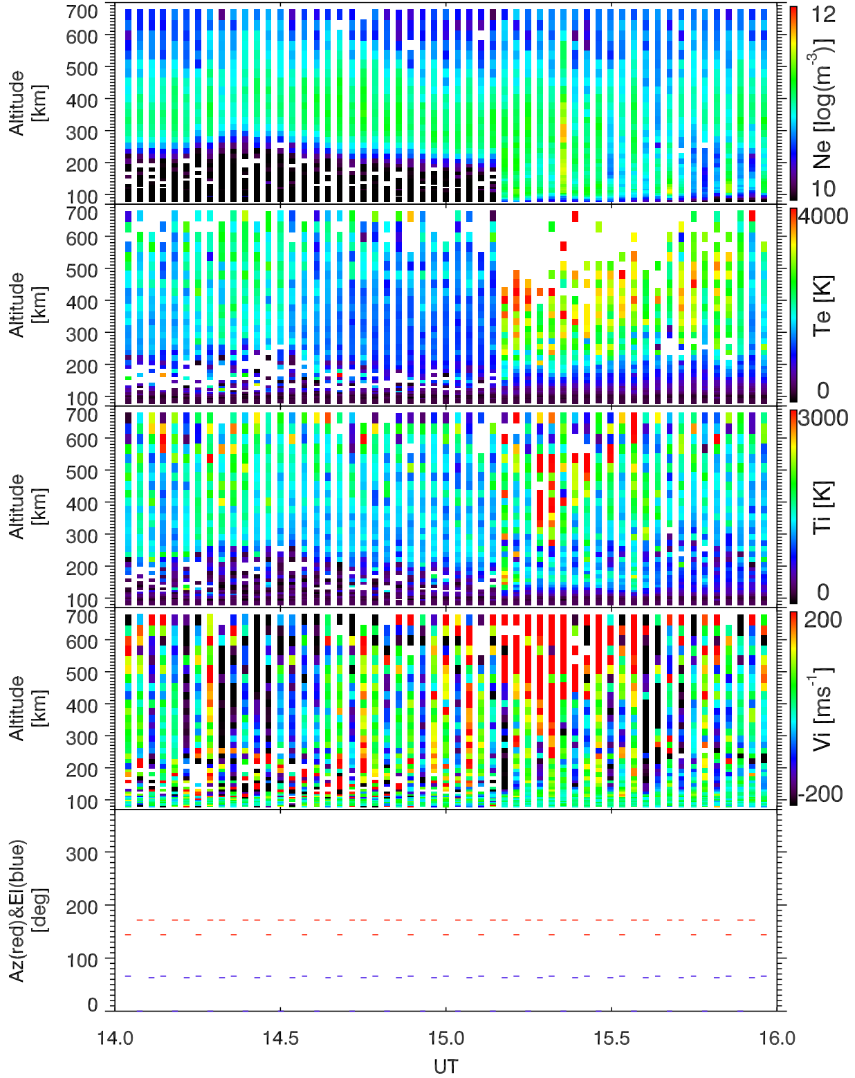
EISCAT 2003-11-16_14_16UT_steffe_ant@32m.
