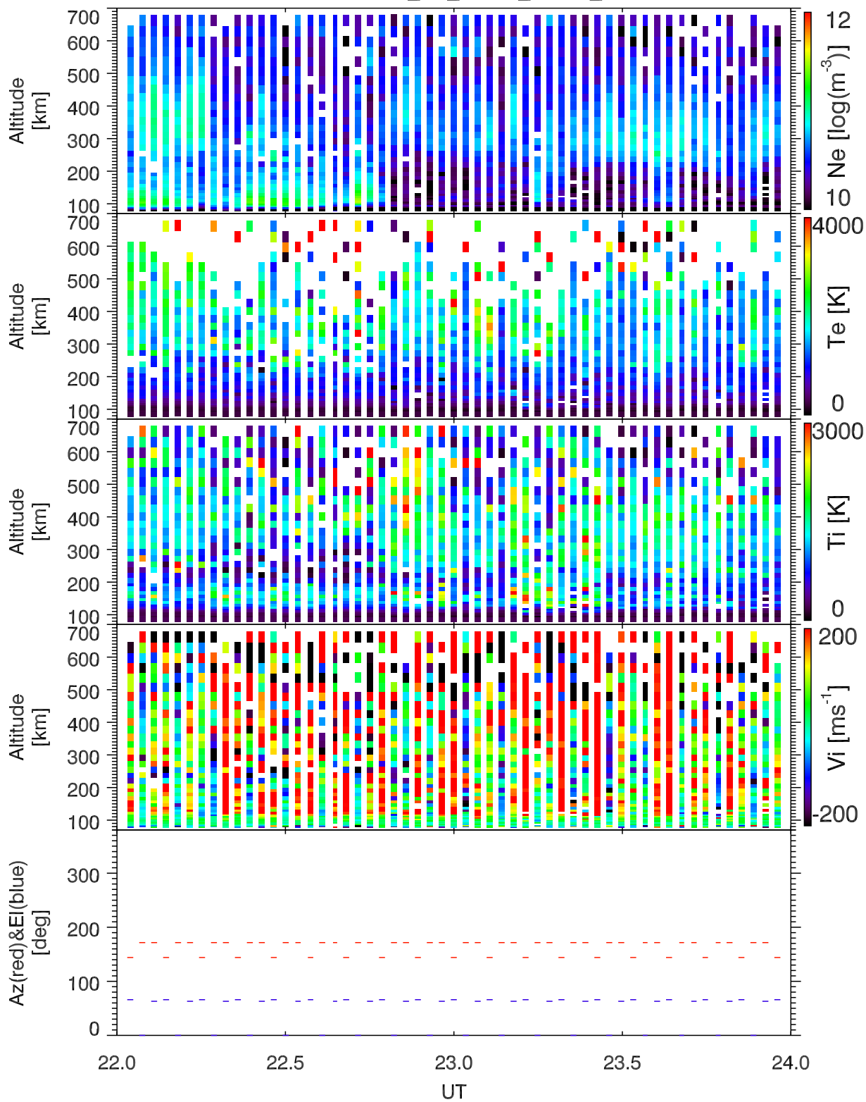
EISCAT 2003-11-16_22_24UT_steffe_ant@32m.
