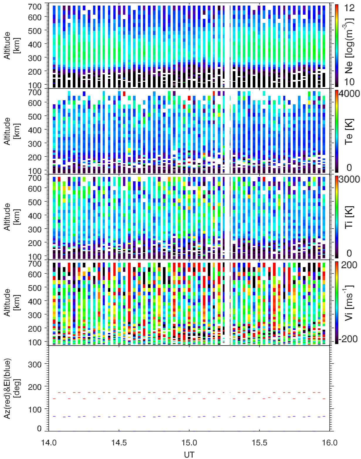
EISCAT 2003-11-17_14_16UT_steffe_ant@32m.
