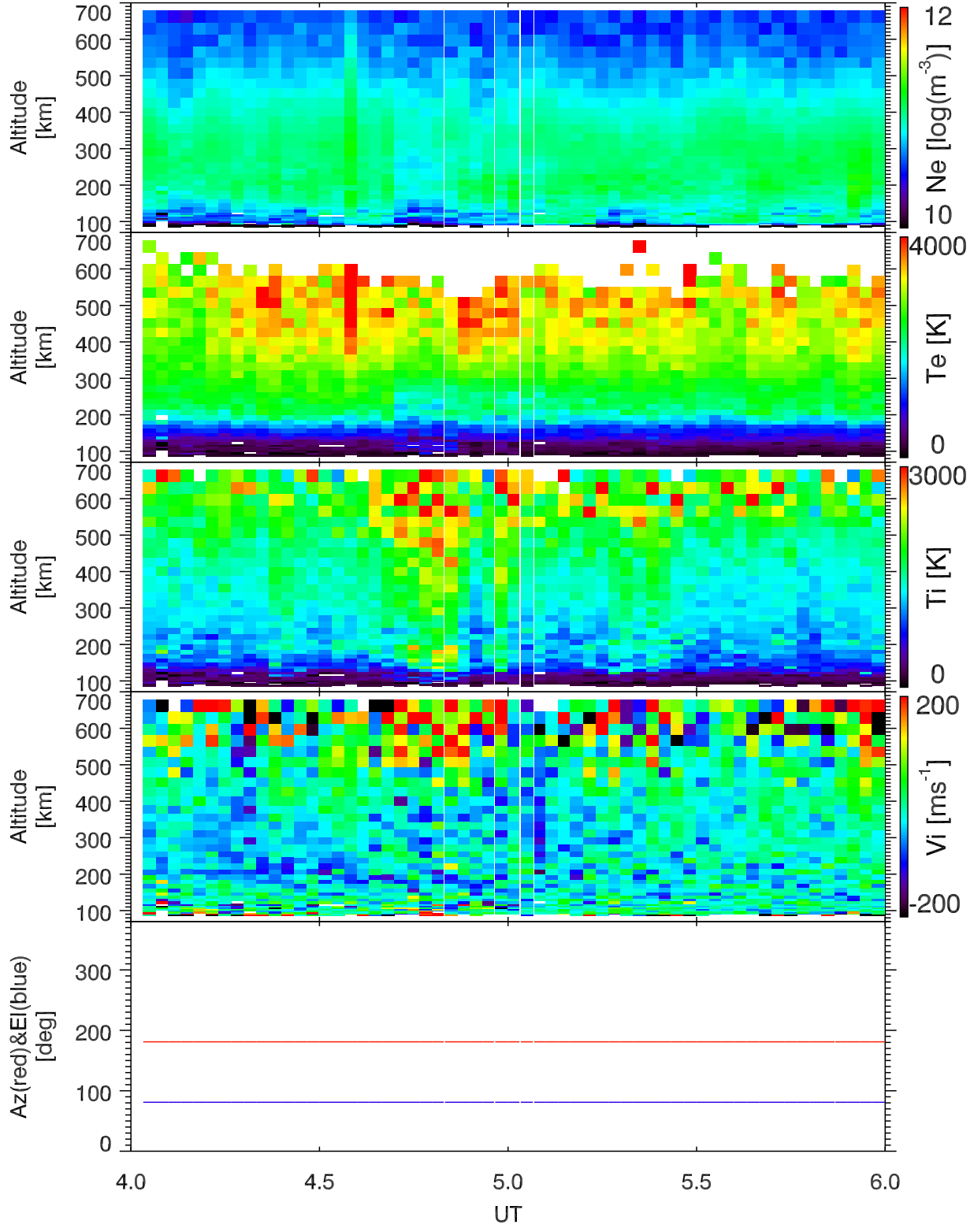
EISCAT 2004-06-03_04_06UT_tau0_120@42m.
