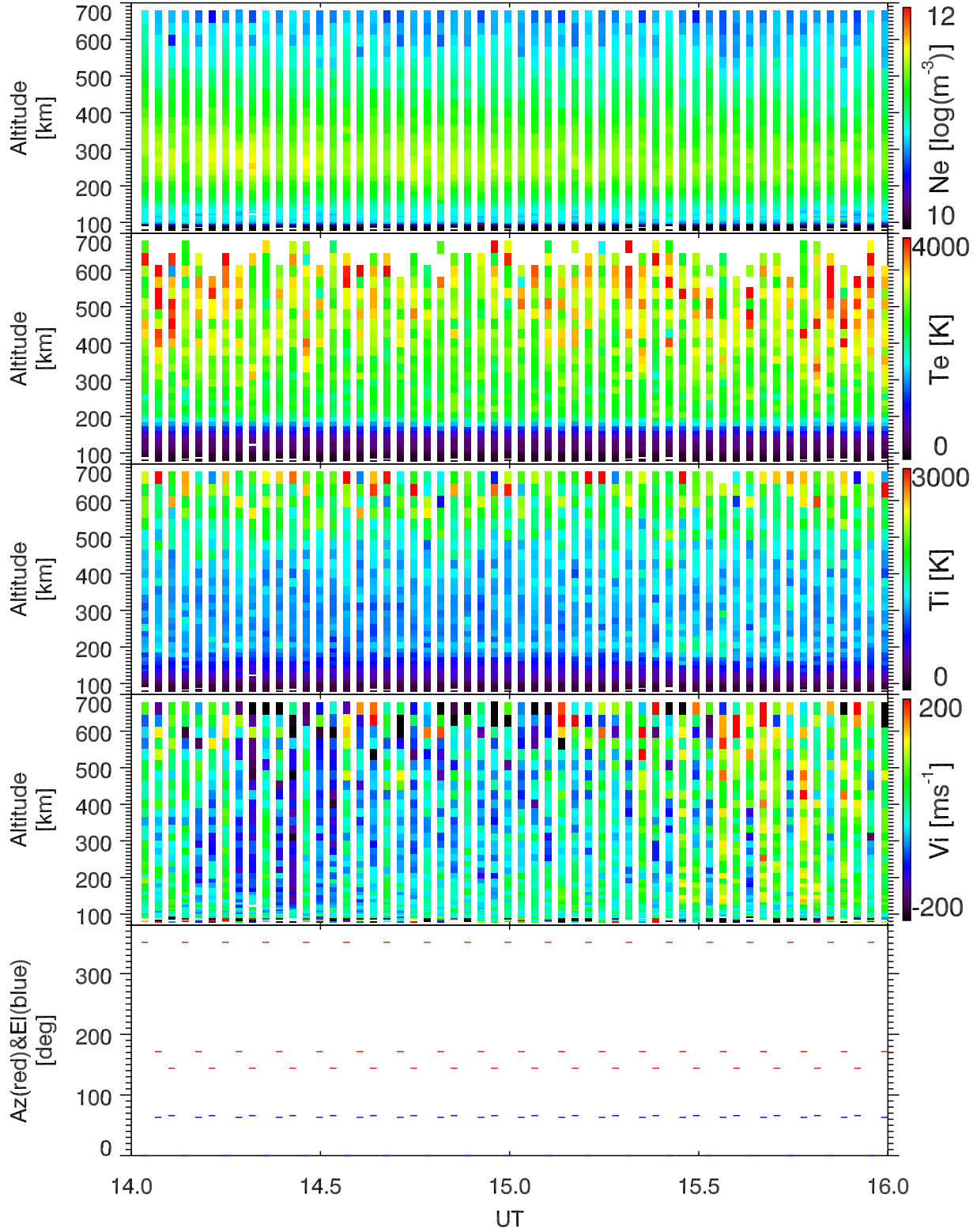
EISCAT 2004-06-05_14_16UT_steffe_ant@32m.
