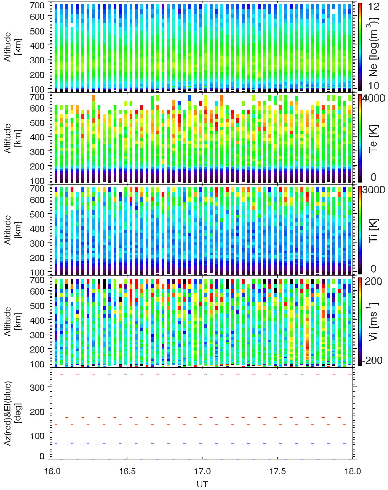
EISCAT 2004-06-06_16_18UT_steffe_ant@32m.
