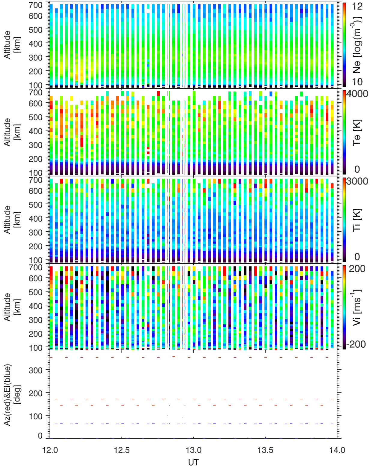
EISCAT 2004-06-07_12_14UT_steffe_ant@32m.
