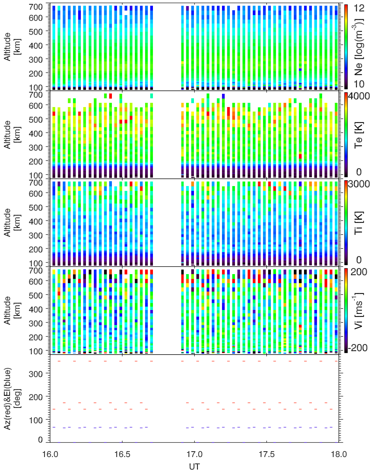
EISCAT 2004-06-07_16_18UT_steffe_ant@32m.
