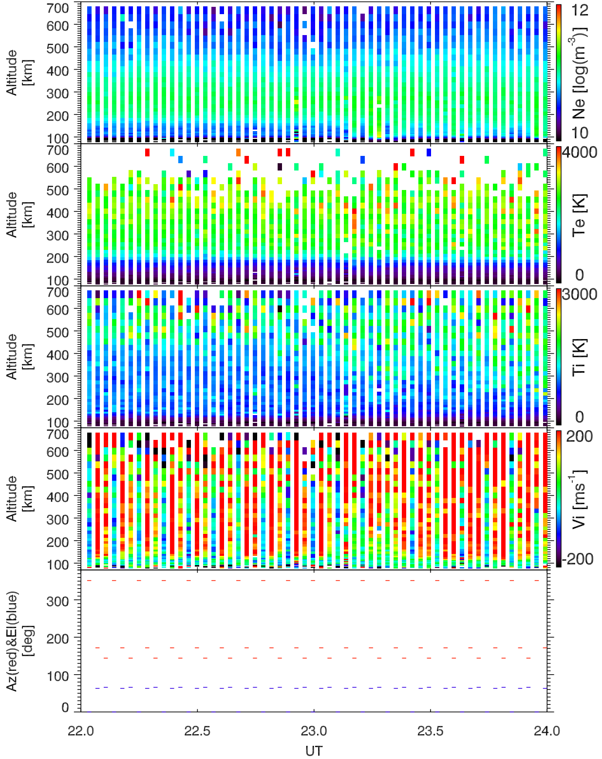
EISCAT 2004-06-07_22_24UT_steffe_ant@32m.
