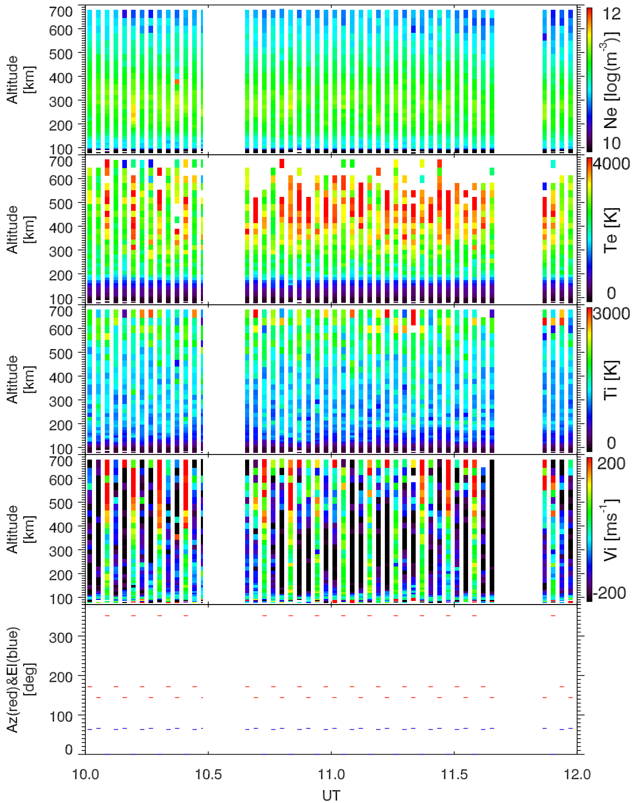
EISCAT 2004-06-08_10_12UT_steffe_ant@32m.
