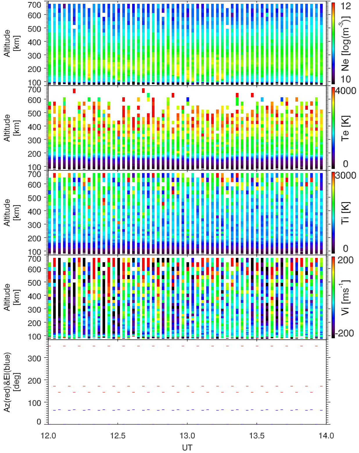
EISCAT 2004-06-09_12_14UT_steffe_ant@32m.
