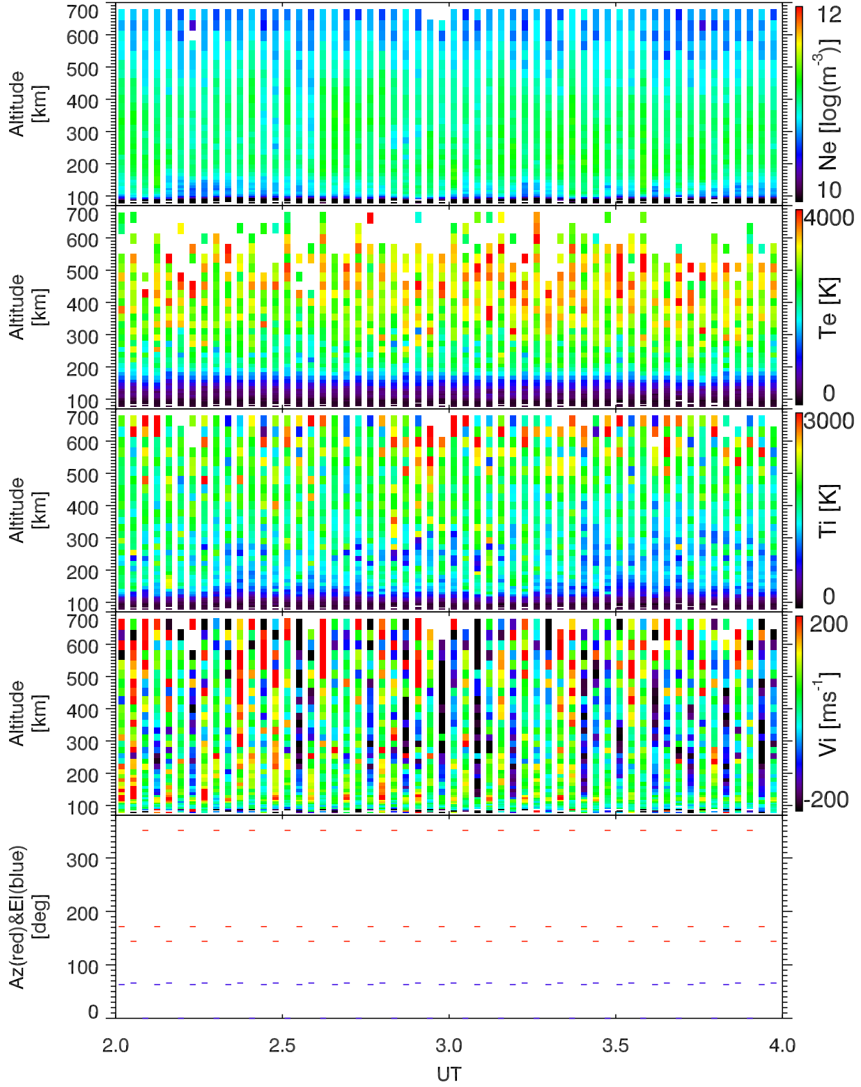
EISCAT 2004-06-10_02_04UT_steffe_ant@32m.
