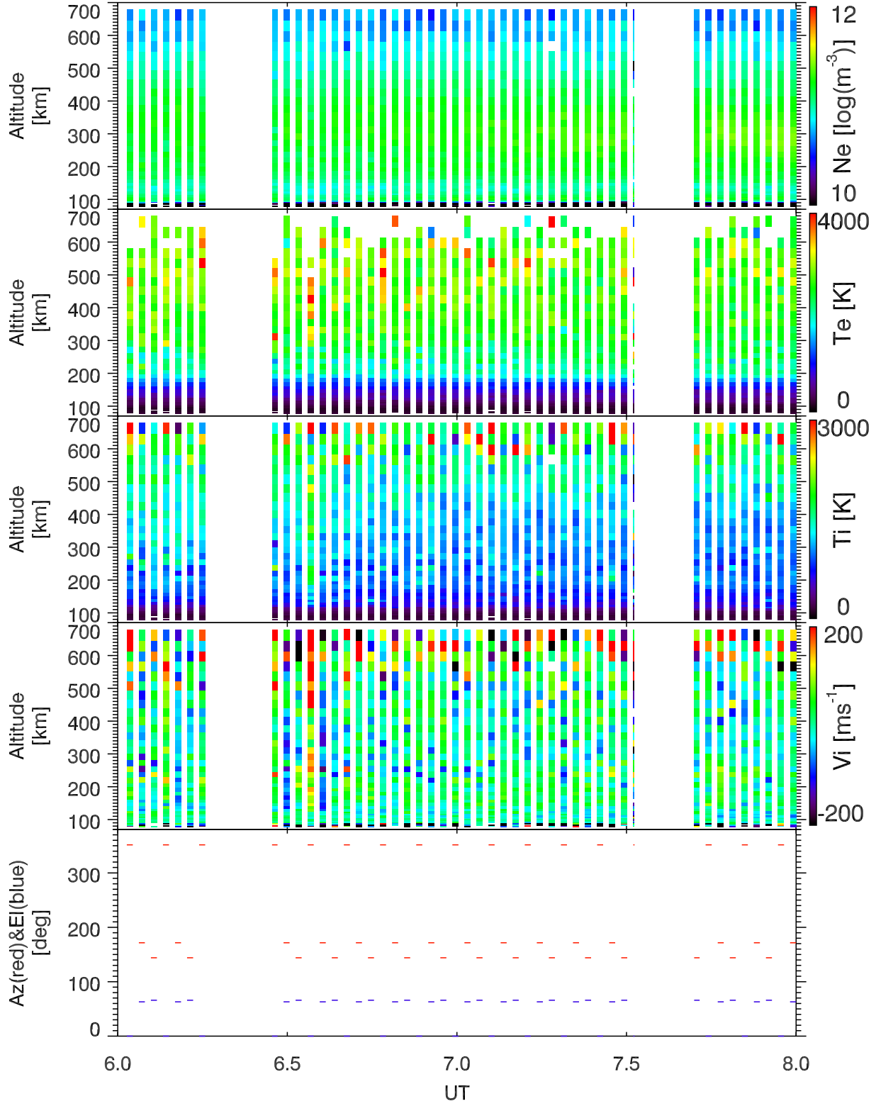
EISCAT 2004-06-10_06_08UT_steffe_ant@32m.
