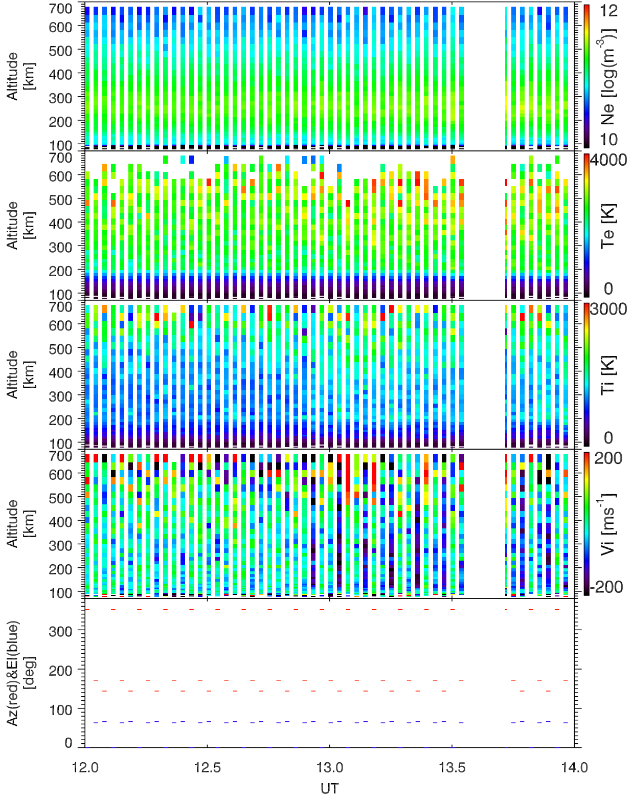
EISCAT 2004-06-10_12_14UT_steffe_ant@32m.
