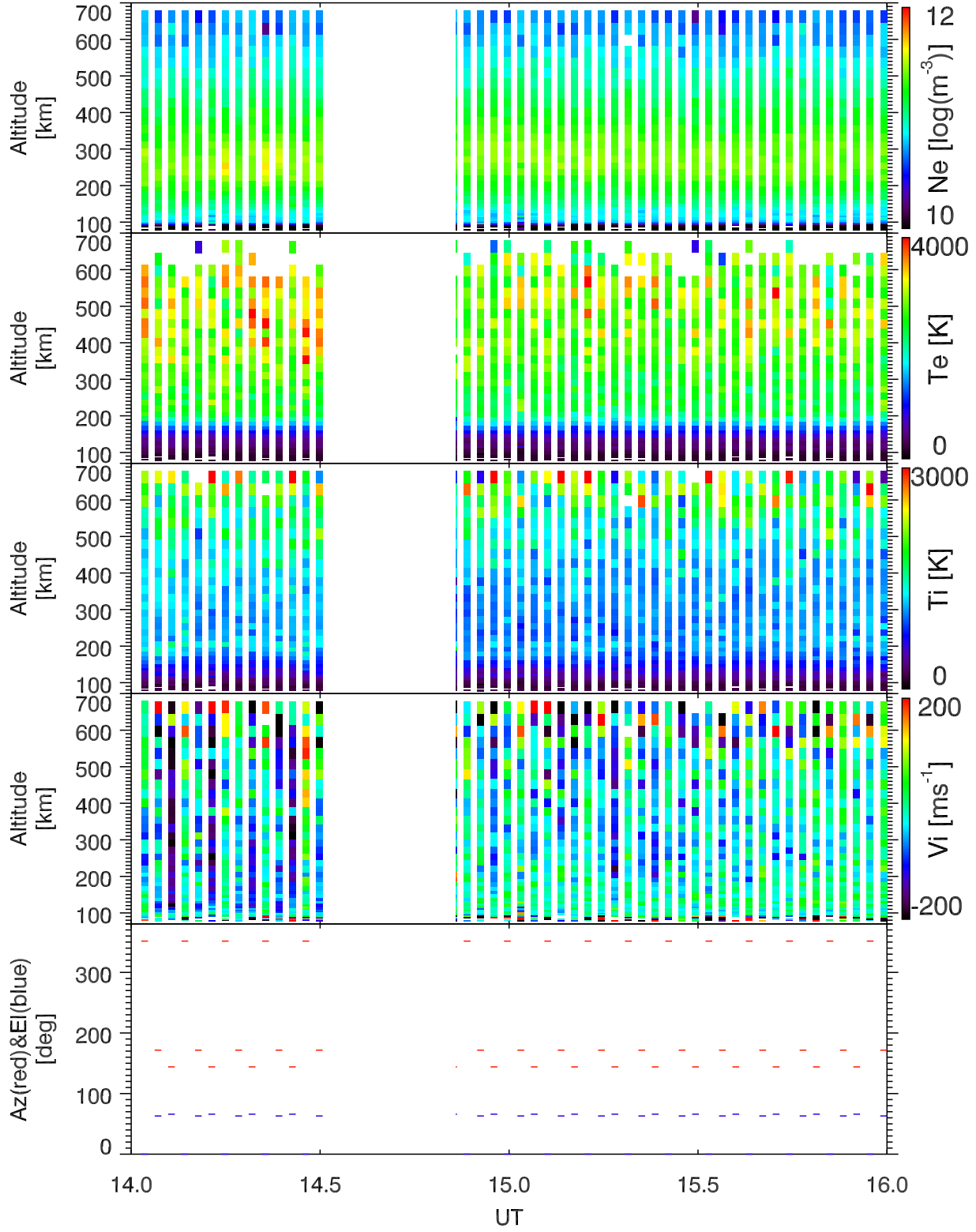
EISCAT 2004-06-10_14_16UT_steffe_ant@32m.
