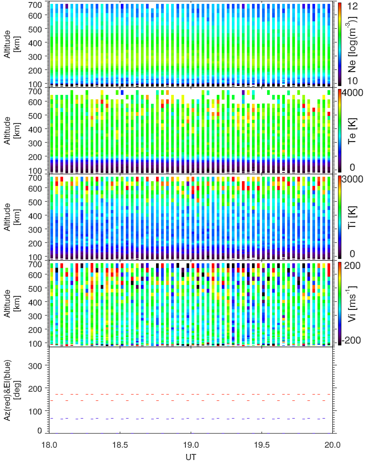
EISCAT 2004-06-13_18_20UT_steffe_ant@32m.
