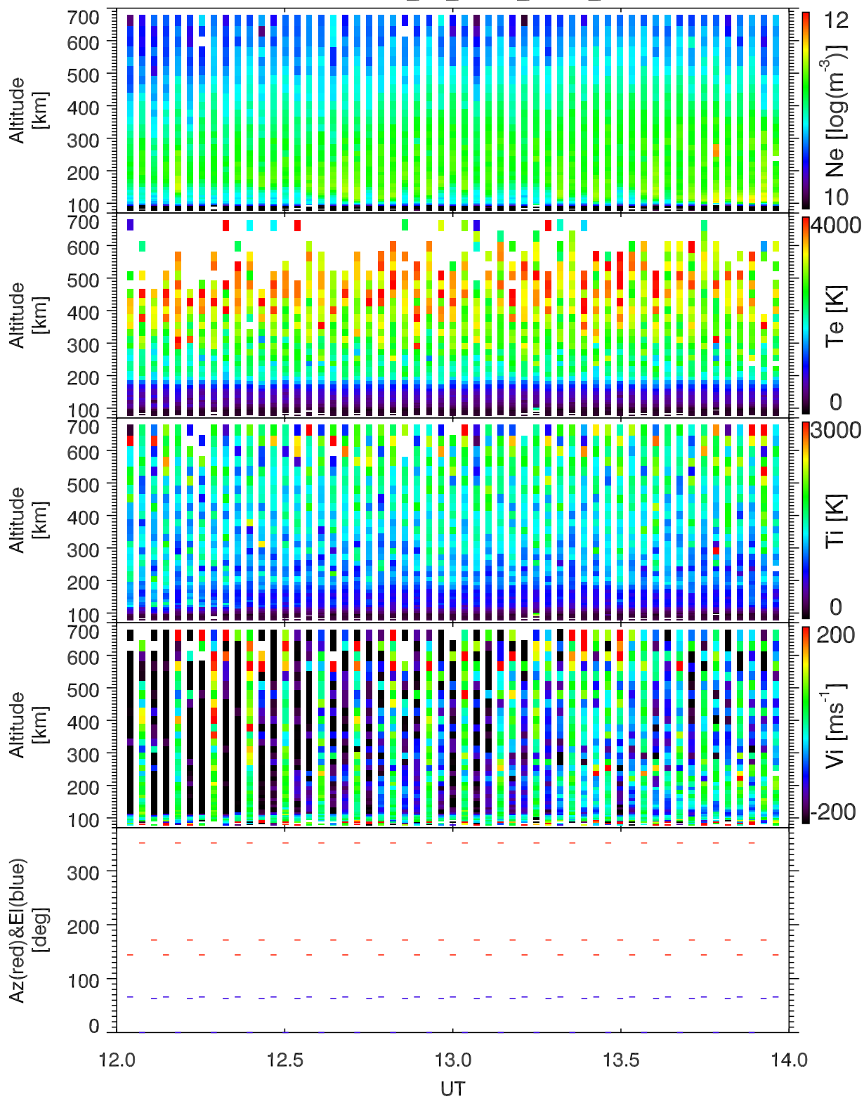
EISCAT 2005-06-13_12_14UT_steffe_ant@32m.
