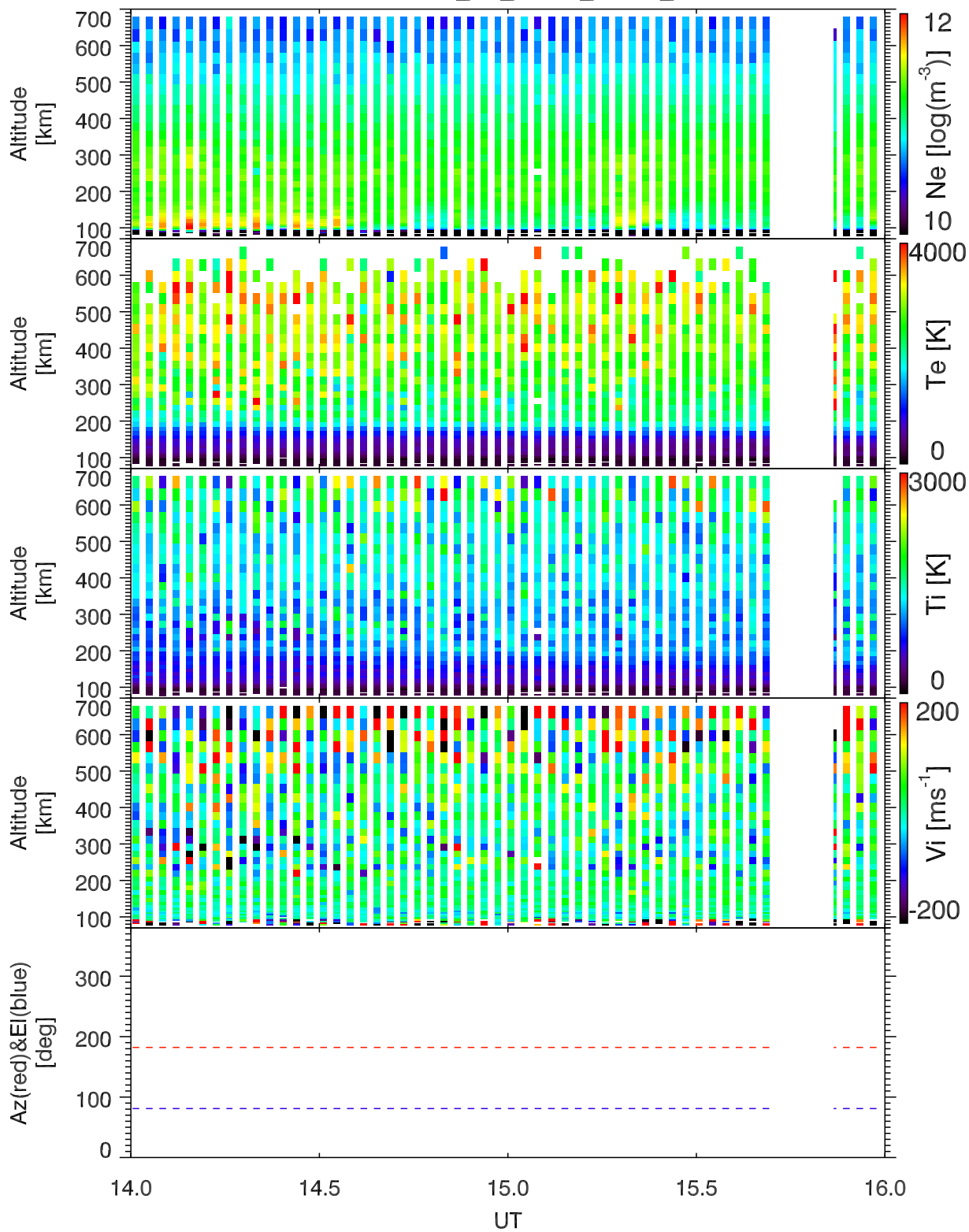
EISCAT 2005-06-13_14_16UT_steffe_ant@42m.
