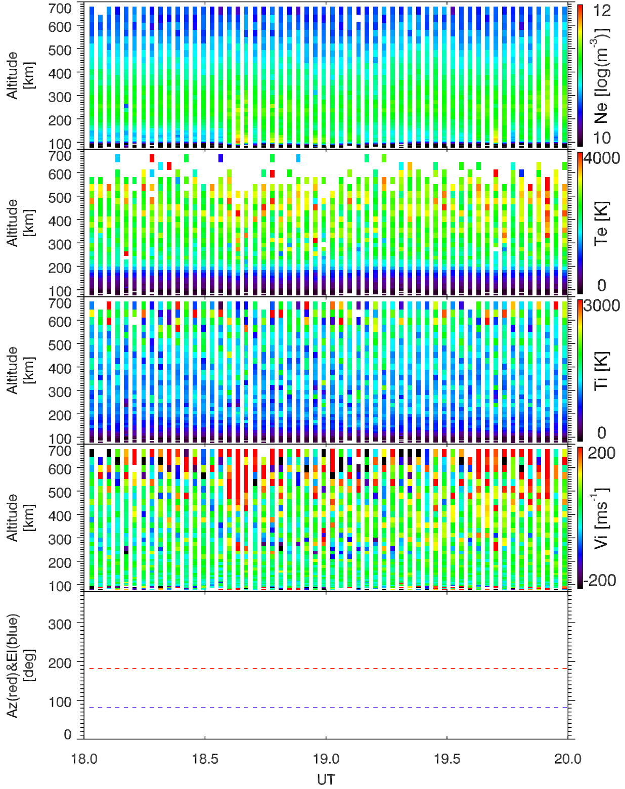
EISCAT 2005-06-13_18_20UT_steffe_ant@42m.
