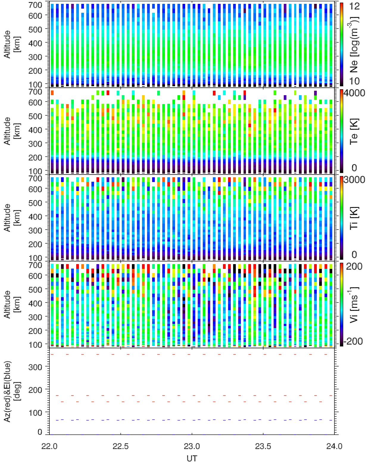
EISCAT 2005-06-15_22_24UT_steffe_ant@32m.
