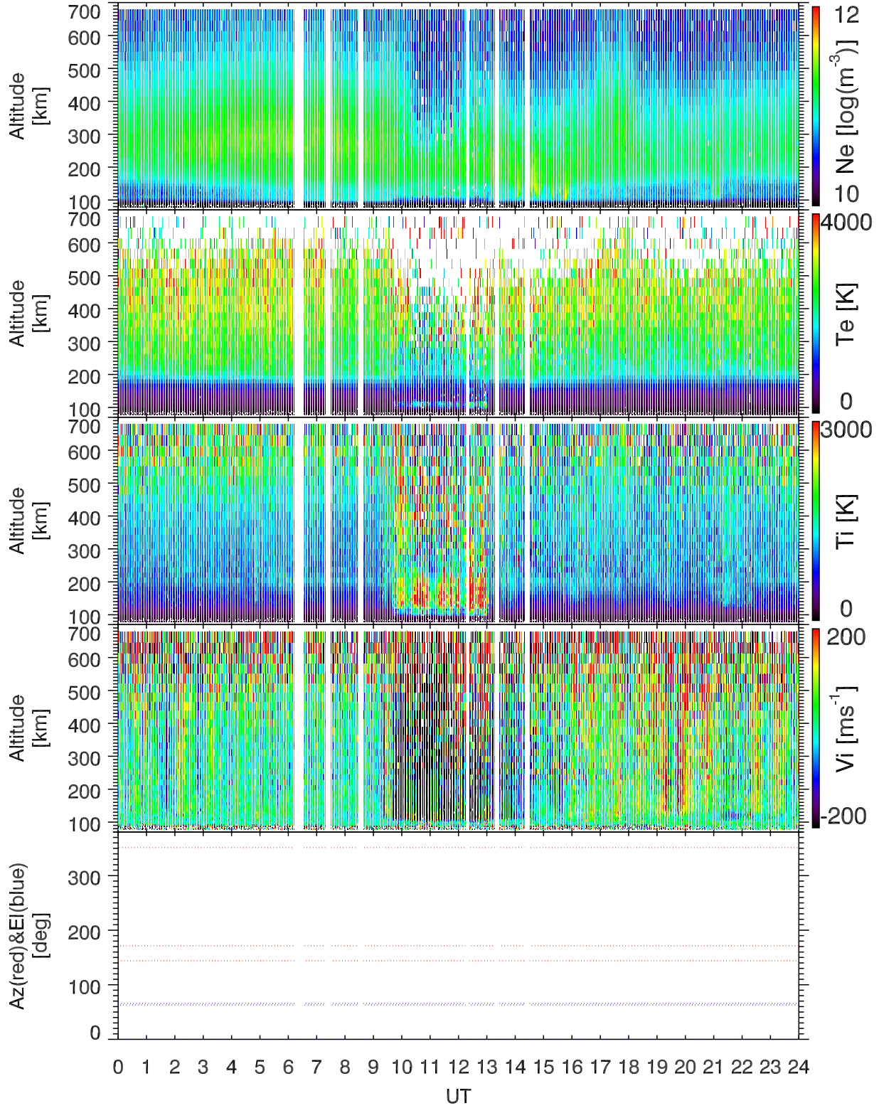
EISCAT 2005-06-16_00_24UT_steffe_ant@32m.
