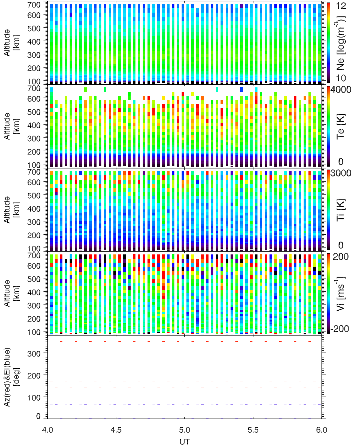
EISCAT 2005-06-16_04_06UT_steffe_ant@32m.
