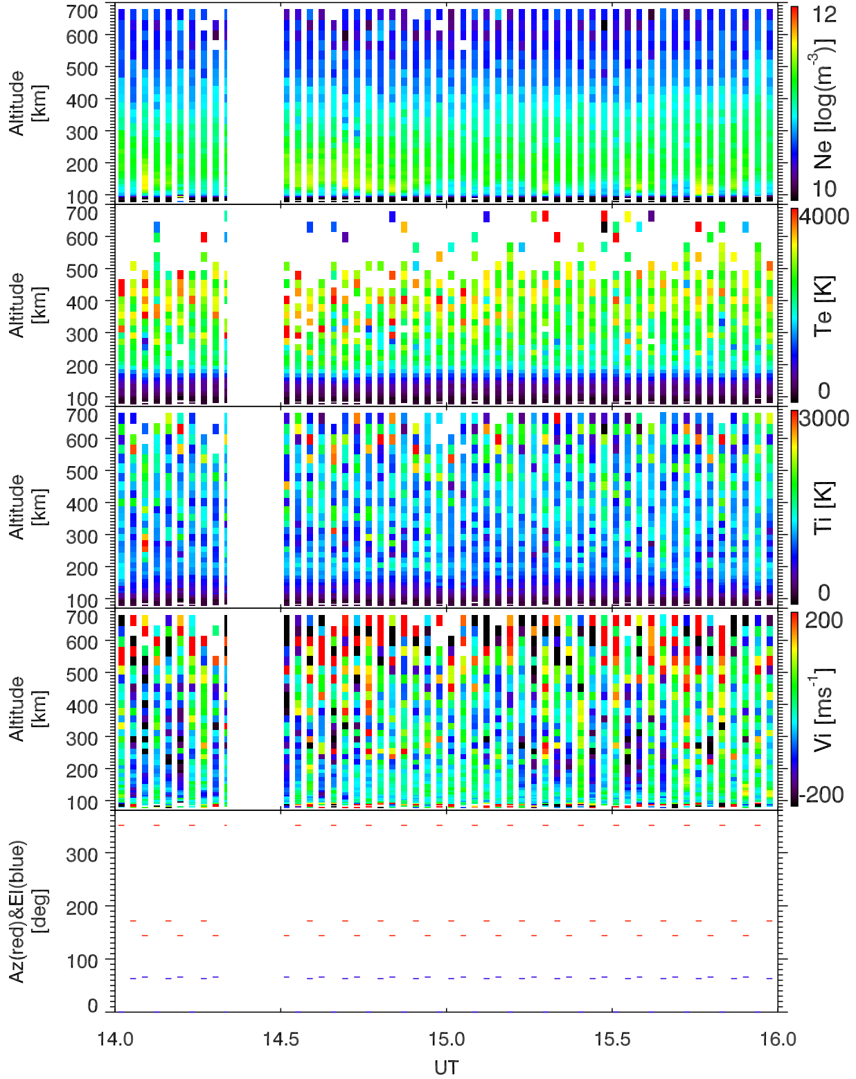
EISCAT 2005-06-16_14_16UT_steffe_ant@32m.
