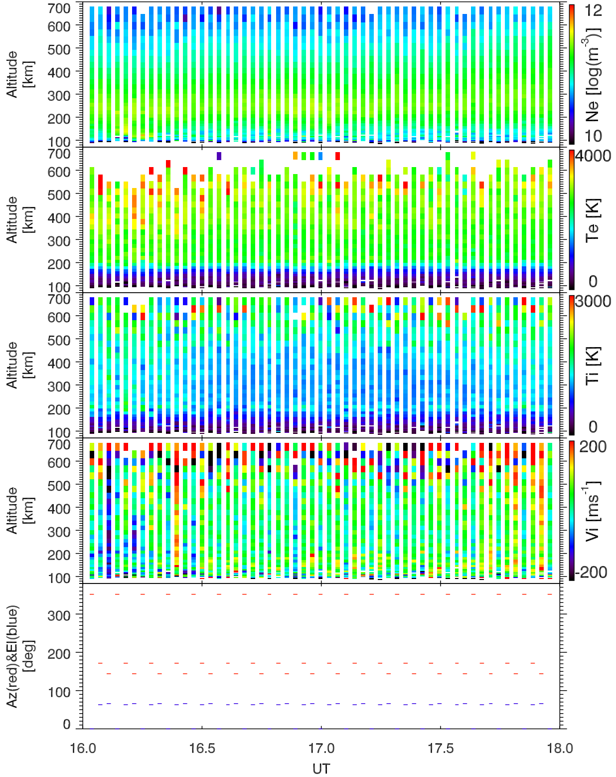
EISCAT 2005-07-01_16_18UT_tau0_ant@32m.
