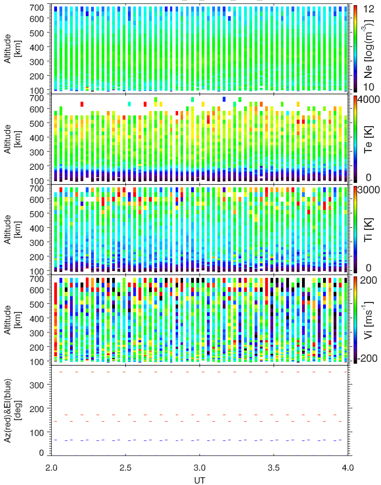
EISCAT 2005-07-02_02_04UT_tau0_ant@32m.
