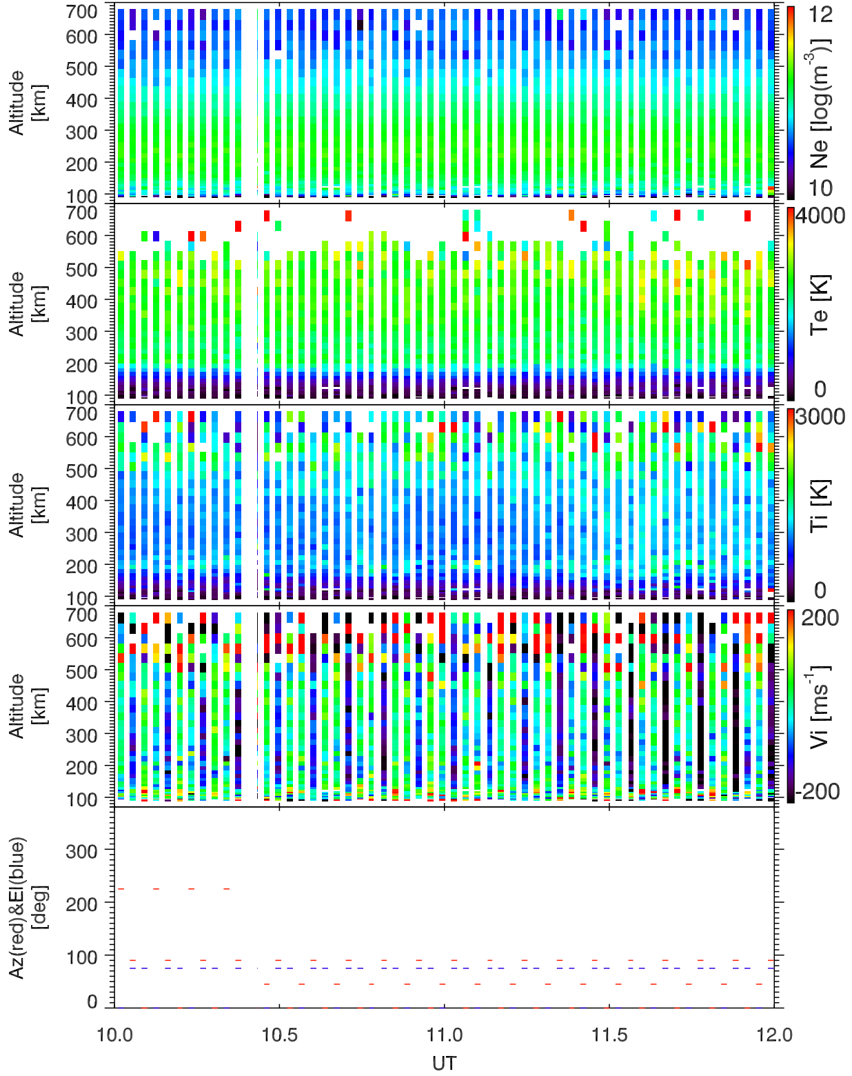
EISCAT 2005-07-23_10_12UT_tau0_ant@32m.
