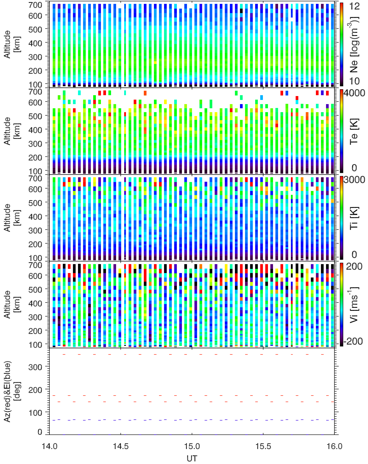
EISCAT 2005-09-01_14_16UT_steffe_ant@32m.
