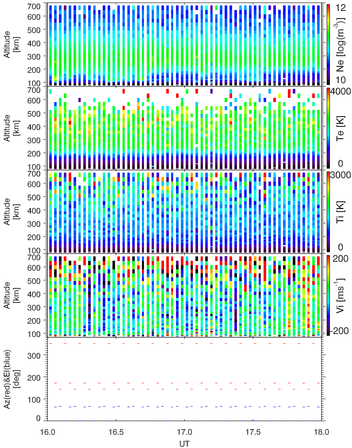
EISCAT 2005-09-03_16_18UT_steffe_ant@32m.
