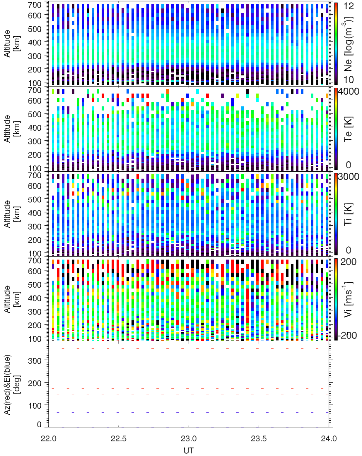
EISCAT 2005-09-03_22_24UT_steffe_ant@32m.
