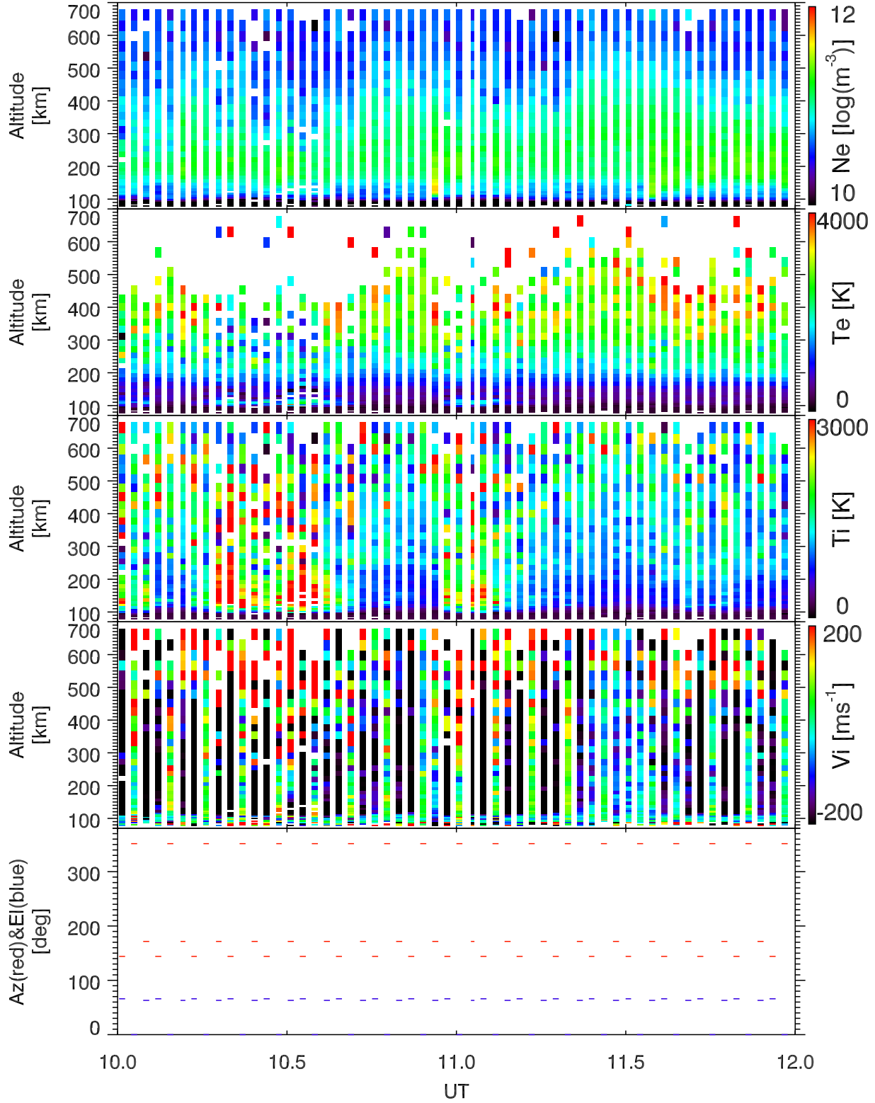
EISCAT 2005-09-04_10_12UT_steffe_ant@32m.
