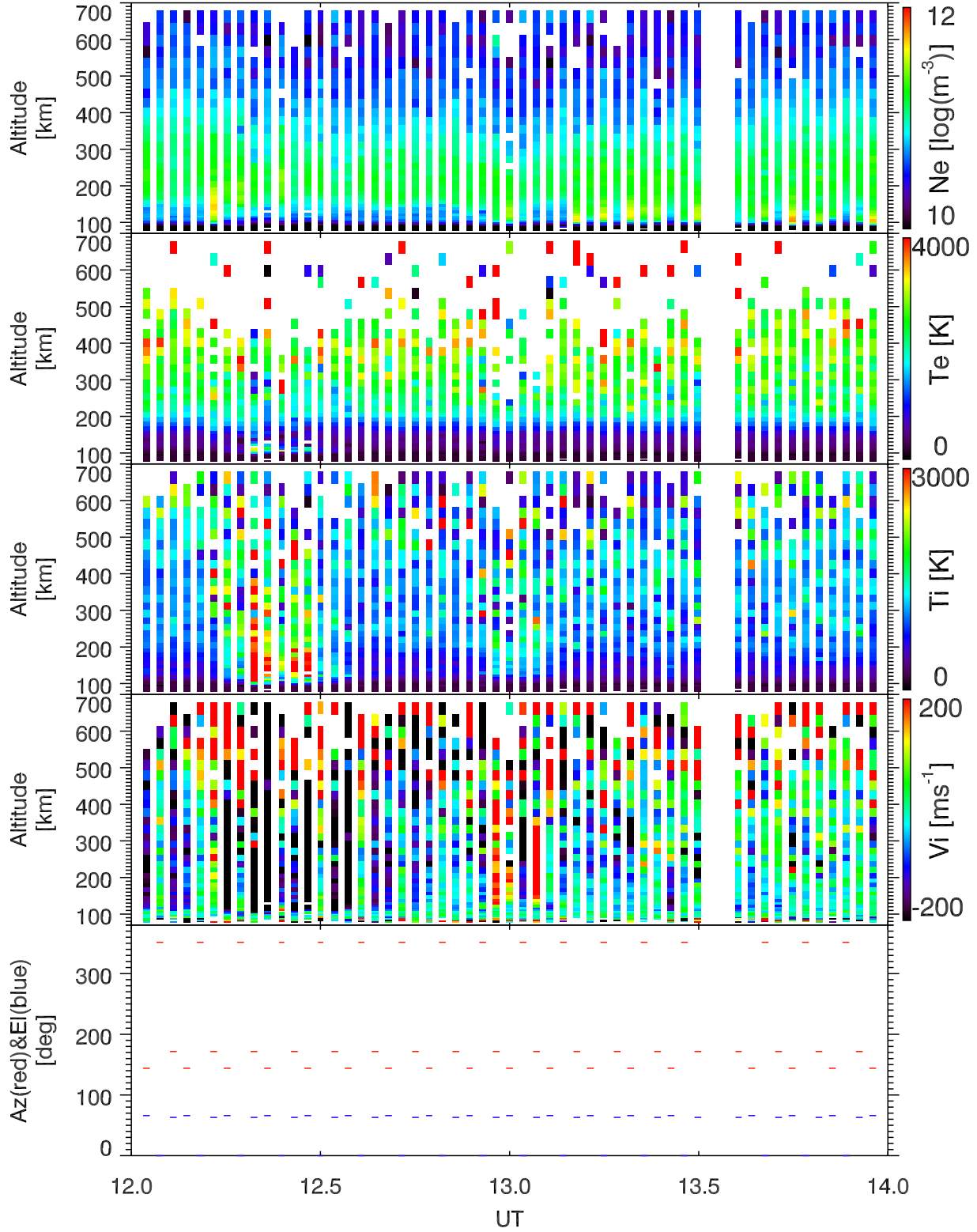
EISCAT 2005-09-04_12_14UT_steffe_ant@32m.
