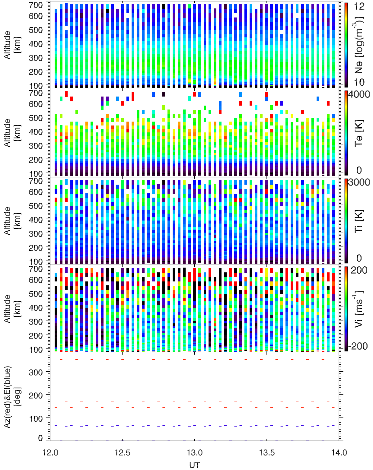
EISCAT 2005-09-05_12_14UT_steffe_ant@32m.
